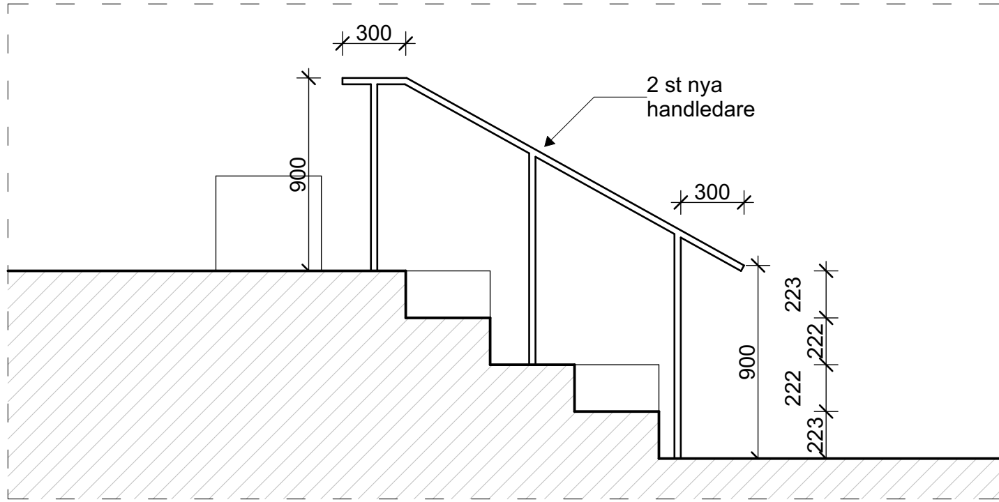
Sektion C-C minigradäng 1:25
