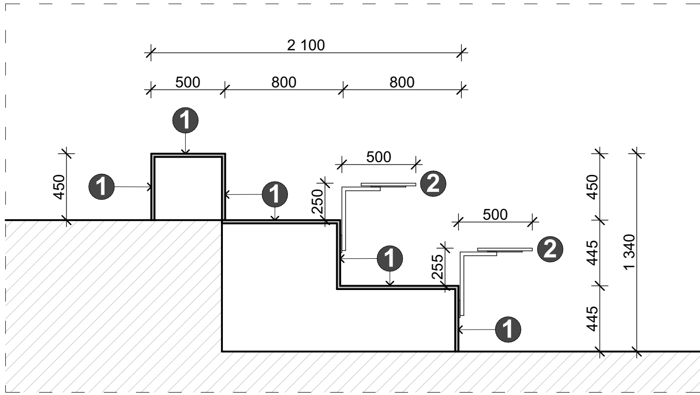
Sektion B-B minigradäng 1:25
