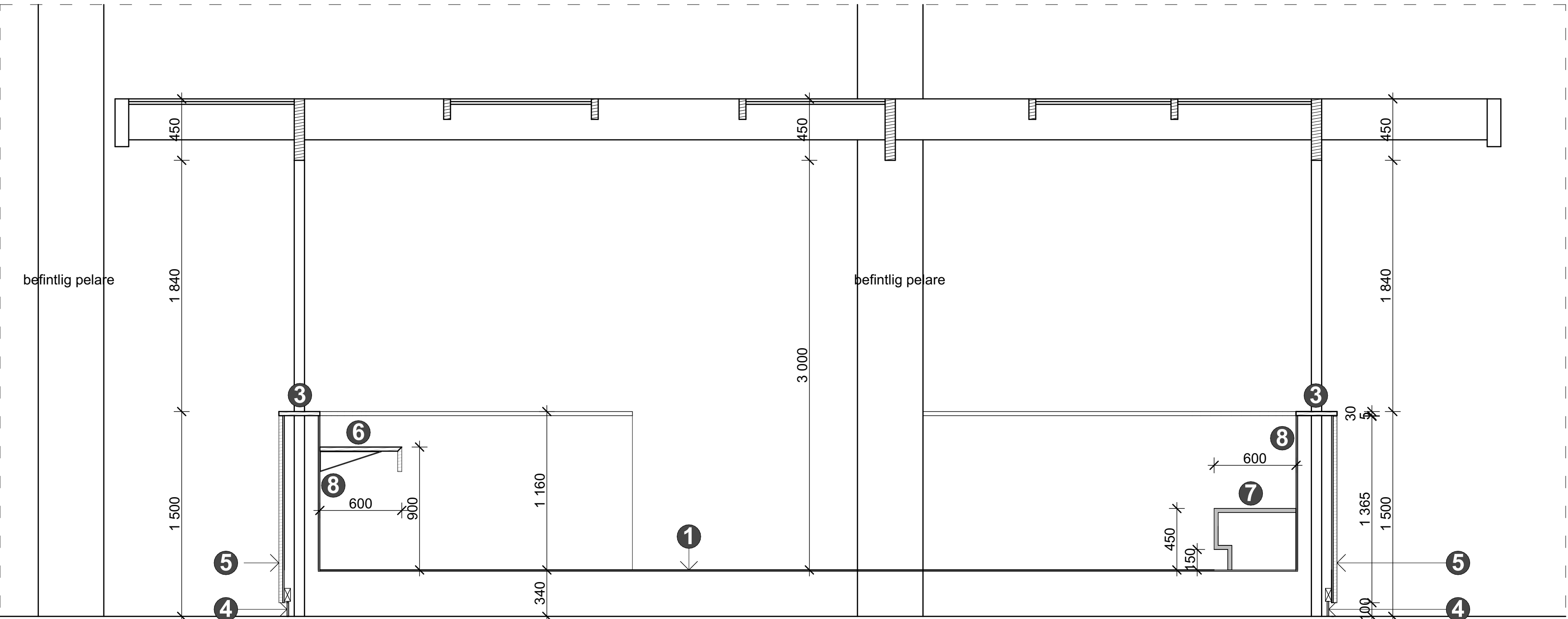
A-A Sektion upphöjd yta 1:25
